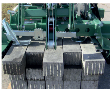
Putere mare de schimb piatră cubică personalizată cu Shifting Adapter-Plus
