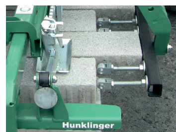
Shifting Adapter-Plus cu Shifting Adapter-Plus chiar pentru cuburi non- standard
