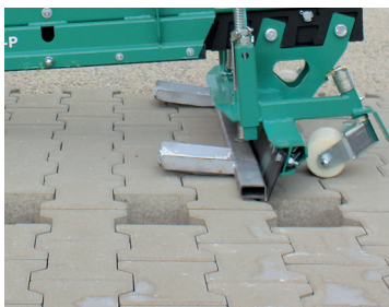
Push-off System Asigură un pavaj de calitate
